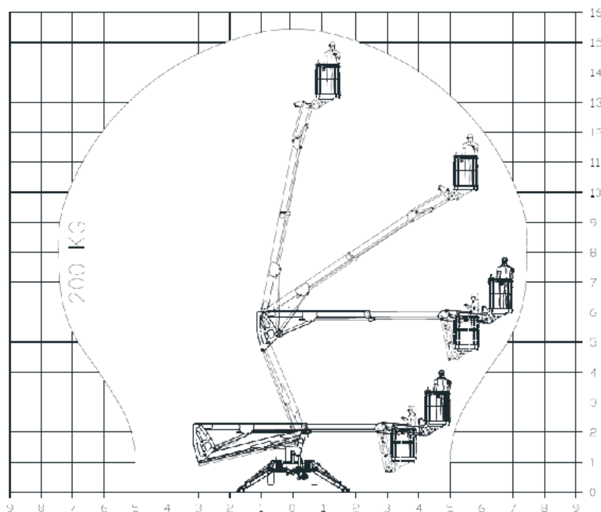
Figur 2. Arbeidsdiagram for TM13G
