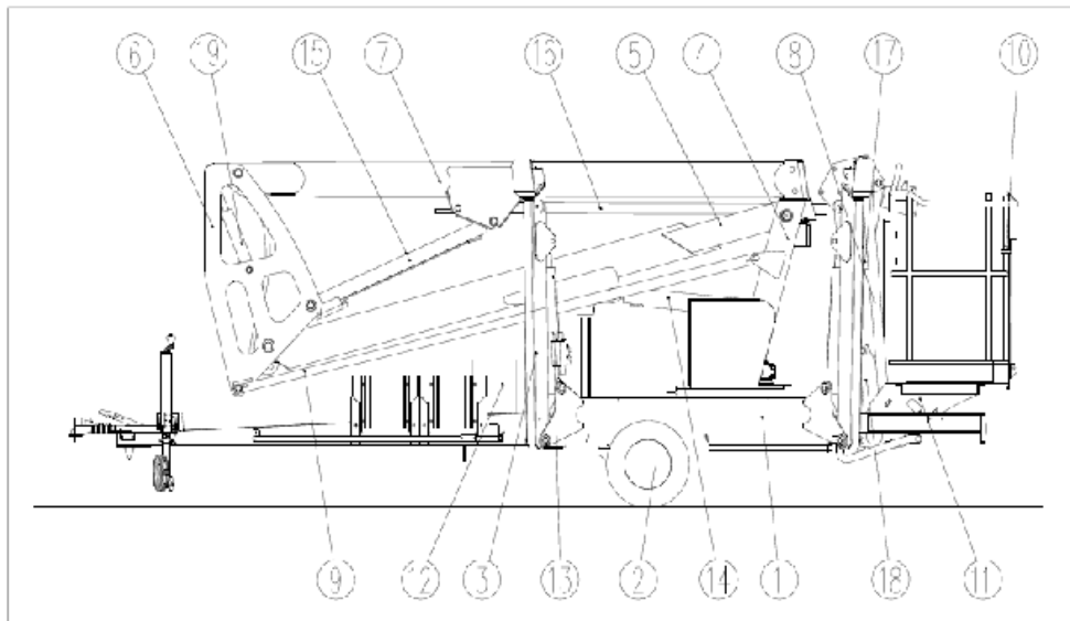
Figur 1. Hoveddelen av den justerbare Europelift TM13G arbeidsplattformen med kurv.
